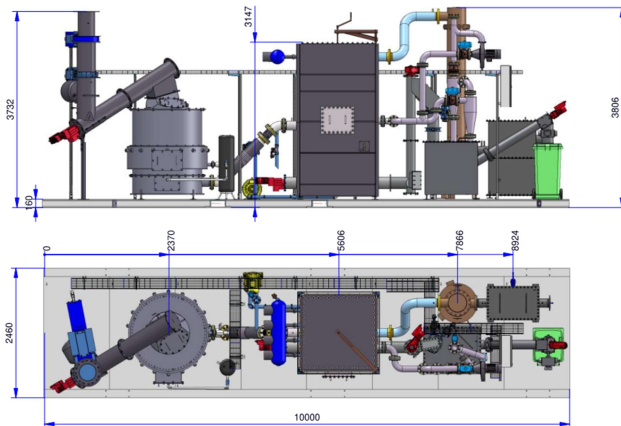
Abbildung: Holzvergaser als Rahmenlösung mit Abmessungen
