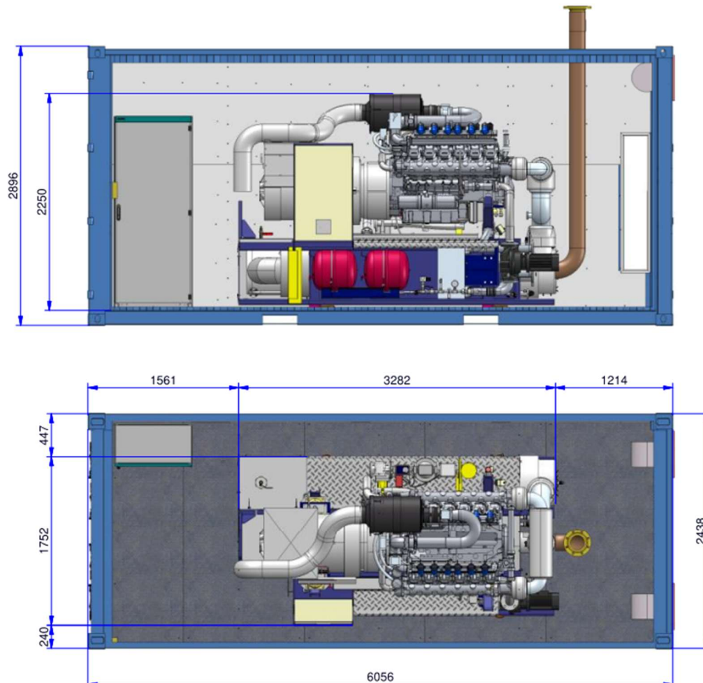
Abbildung: BHKW-Container mit Abmessungen
